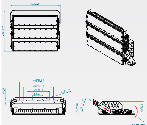
MF-FLL720WB
